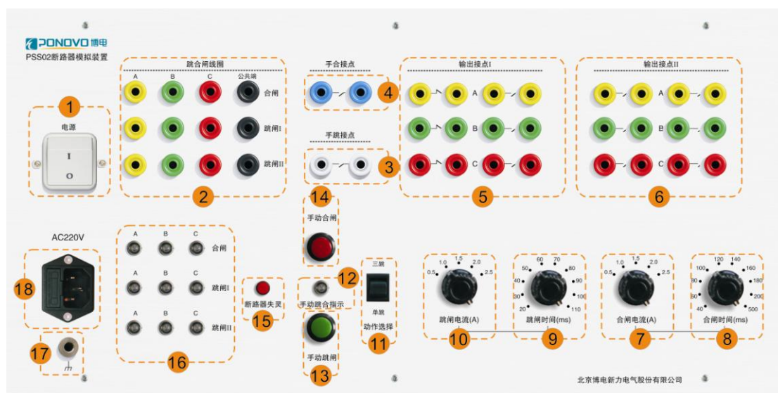
图 1 PSS02、PSS05 断路器模拟装置面板图
