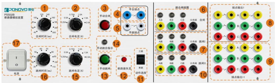
图 2 PSS02B、PSS05B 断路器模拟装置面板图
