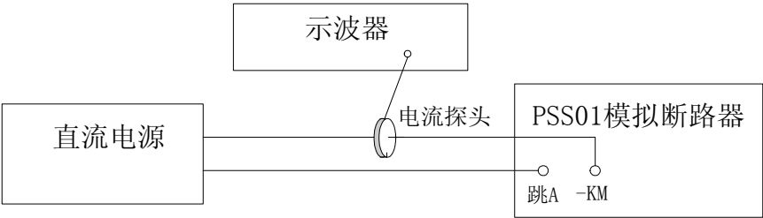
图 8 断路器模拟装置线圈电流值测量示意图
