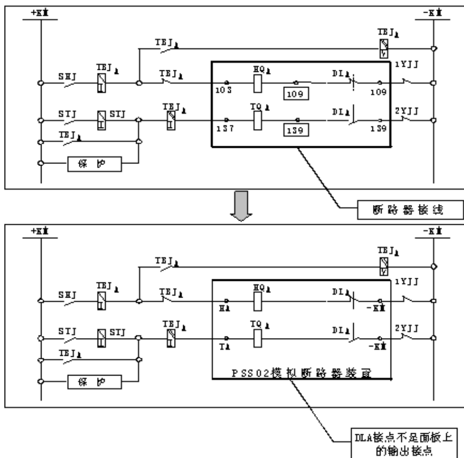
图 5 PSS02 (B/C)、PSS05 (B/C) 接入实际二次回路示意图
