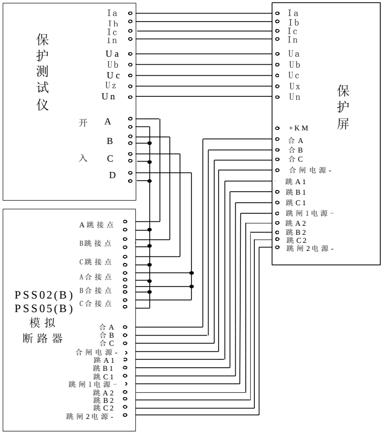
图 4 PSS02(B)、PSS05(B)模拟断路器与保护测试仪配合进行保护装置整组传动试验系统接线图
