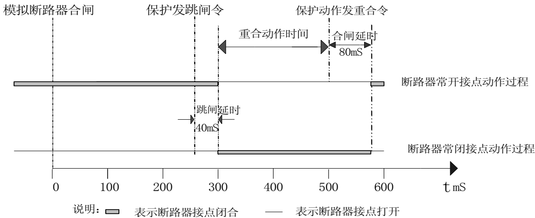
图 7 跳、合闸动作过程示意图
