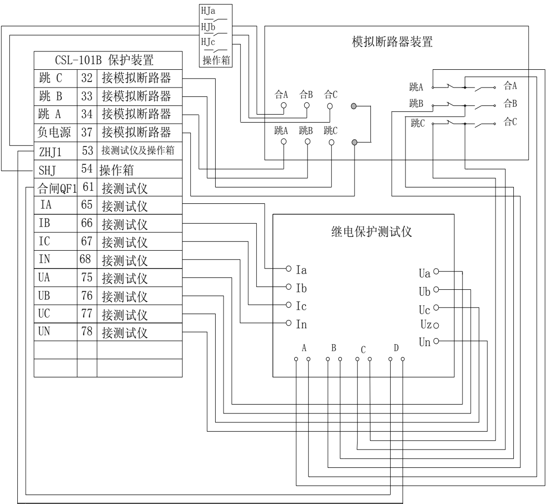
图 6 试验接线
