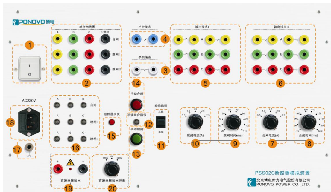
图 3 PSS02C、PSS05C 断路器模拟装置面板图
